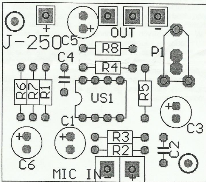
Schemat montażowy
