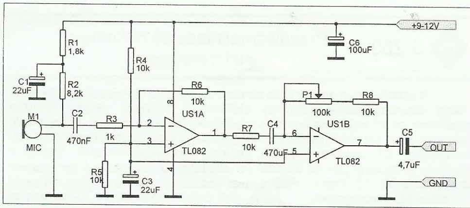
Schemat ideowy
