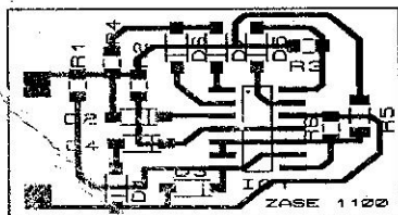
Rozloženie súčiastok
