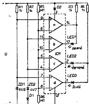
Schéma zapojenia
